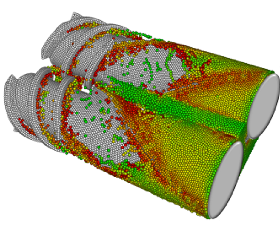
粒子法による樹脂混練機の非定常流動解析
