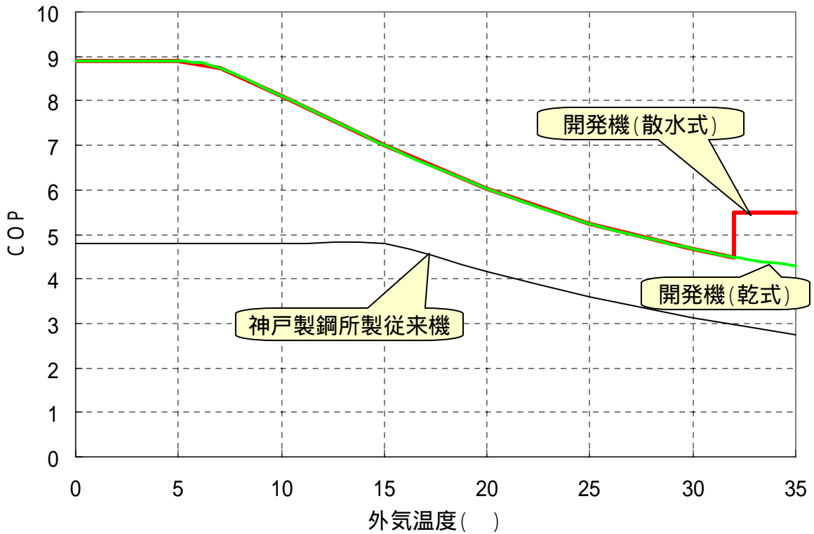
図2. 外気温特性（冷房時）
