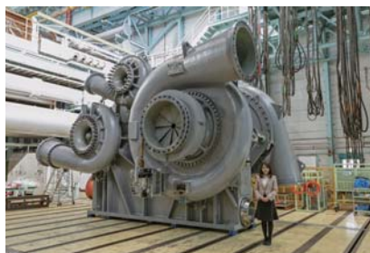
涡机内置涡轮式压缩机
