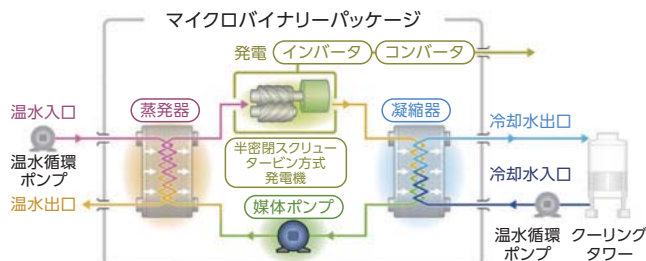
〔バイナリー発電システムによる70kW発電の一例〕
