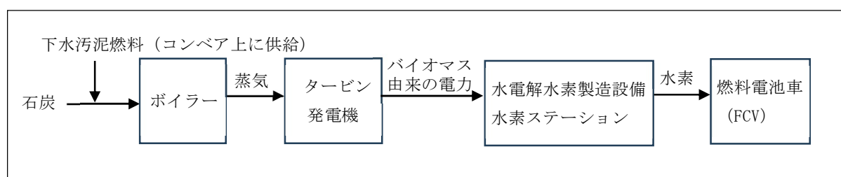
図 4.6-1 下水汚泥燃料を活用した発電システムフロー
