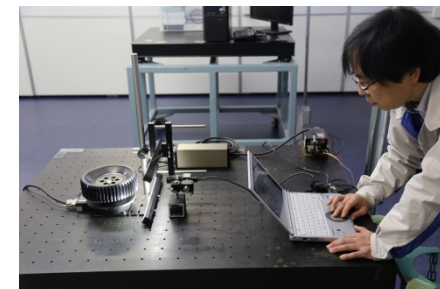
【金型の外観（360度画像）を自動で記録するシステムの試作】
