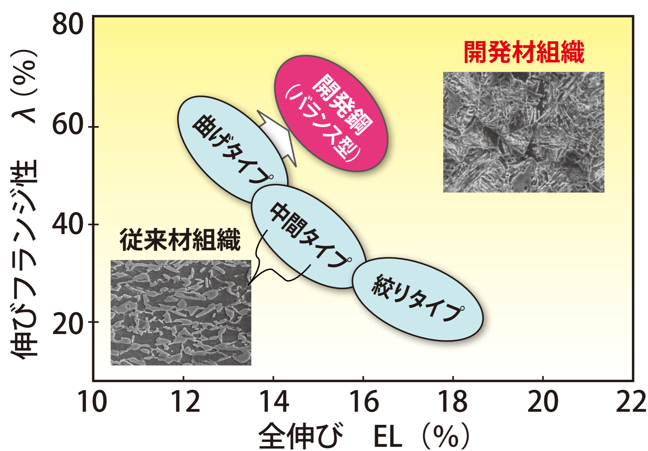
980N/mm 2 級ハイテンのEL-λバランス
