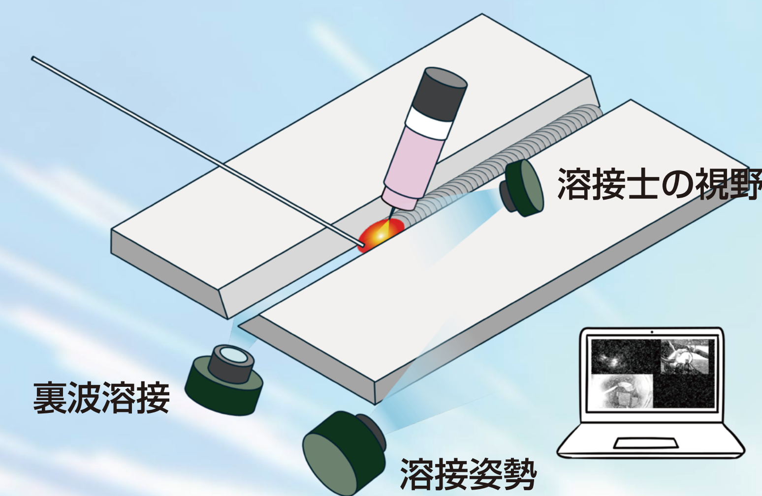
溶接技能向上・継承支援 (技能の見える化)
