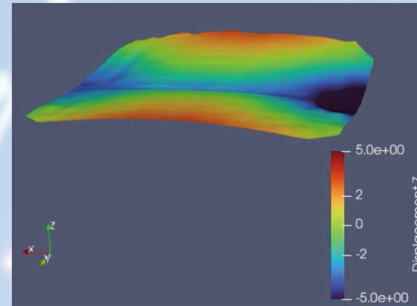
溶接変形測定 (ステレオ画像相関法)
