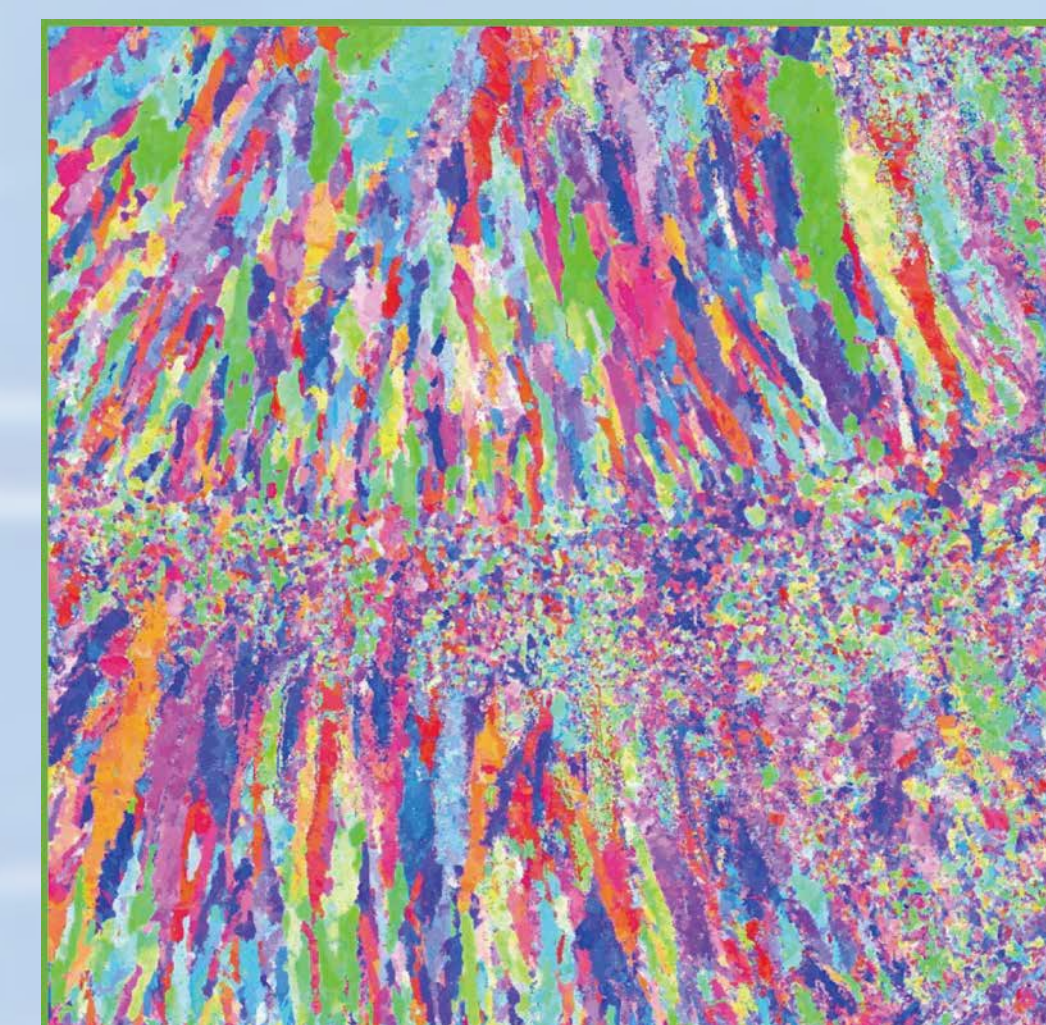
金属組織観察 (EBSD)
