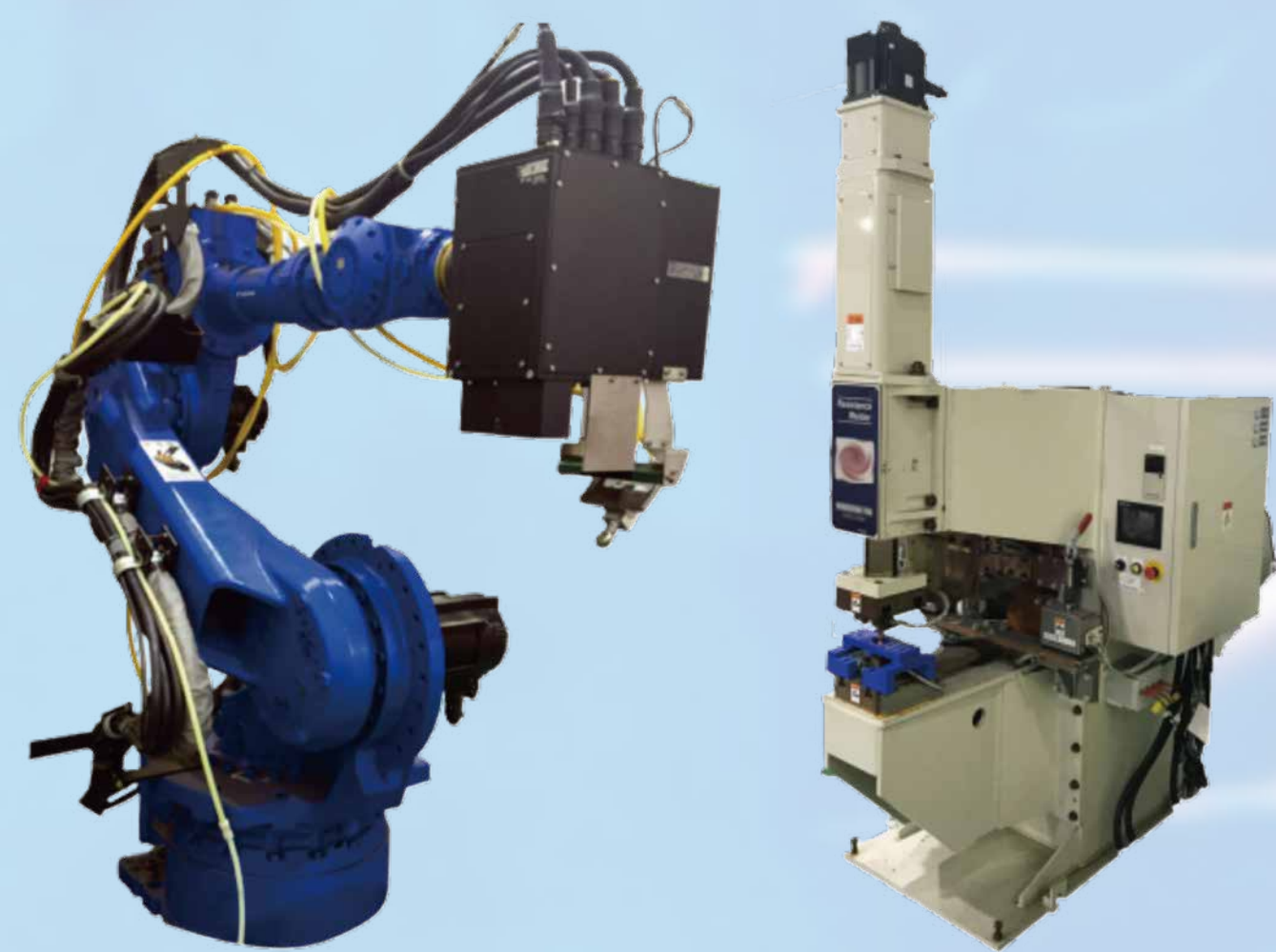
レーザ溶接・スポット溶接
