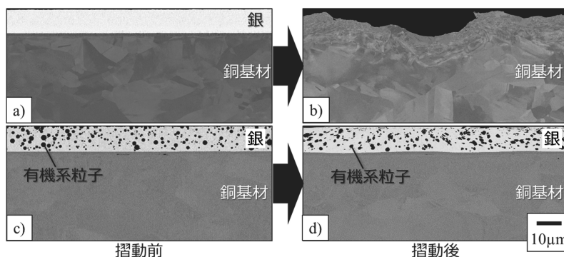
図2 摺動試験前後の断面SEM写真、硬質銀めっき a) 摺動前、b) 摺動後および粒子共析銀めっき c) 摺動前、d) 摺動後
