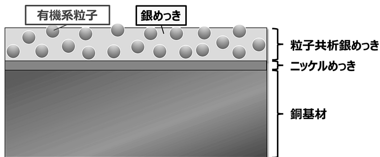
図1 粒子共析銀めっきのめっき構成
