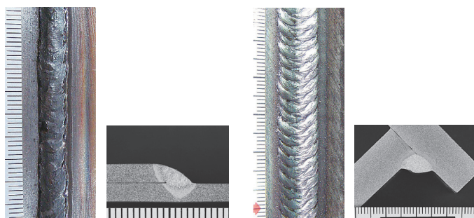
立向下進溶接、板厚3.2mmt (120A-19V、半自動溶接)
