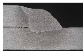
断面マクロ
