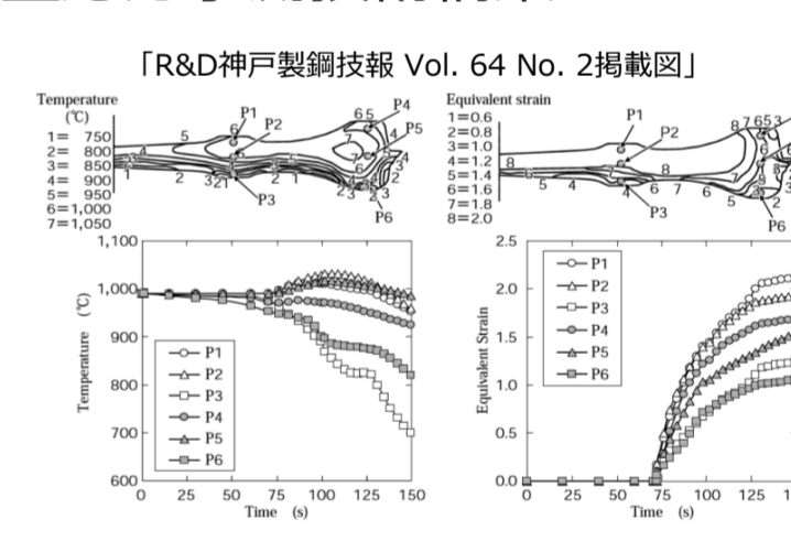
ディスク部品βプロセス鍛造の温度およびひずみ解析結果
