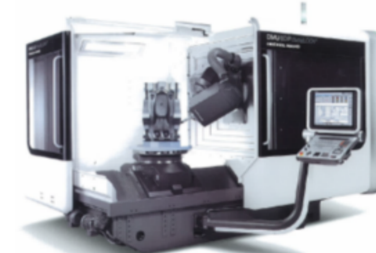
大型5軸同時制御マシニングセンター (DMG-MORI社製 DMU-P100)
