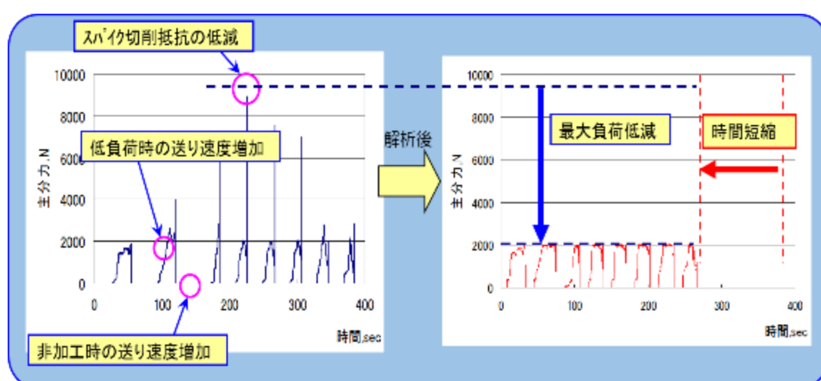
インペラー加工への切削プロセスシミュレーション技術の適用事例 (切削中の負荷の予測結果をもとに、切削送り速度を最適化)
