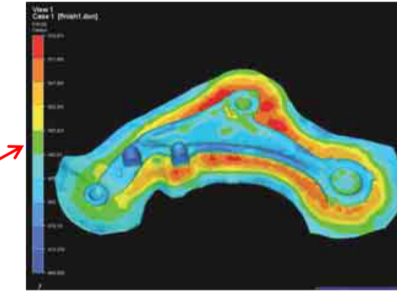
自動車用足廻りサスペンション部材 (鍛造シミュレーション：温度分布)
