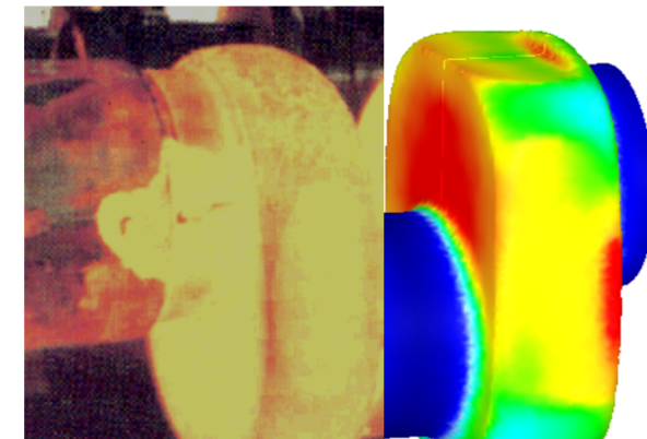
船舶用一体型クランク軸 (RR鍛造シミュレーション：相当ひずみ分布)
