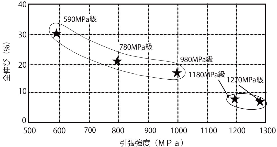
■本鋼板の強度－伸び特性バランスの例
