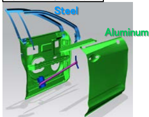
マルチマテリアルドア設計事例
