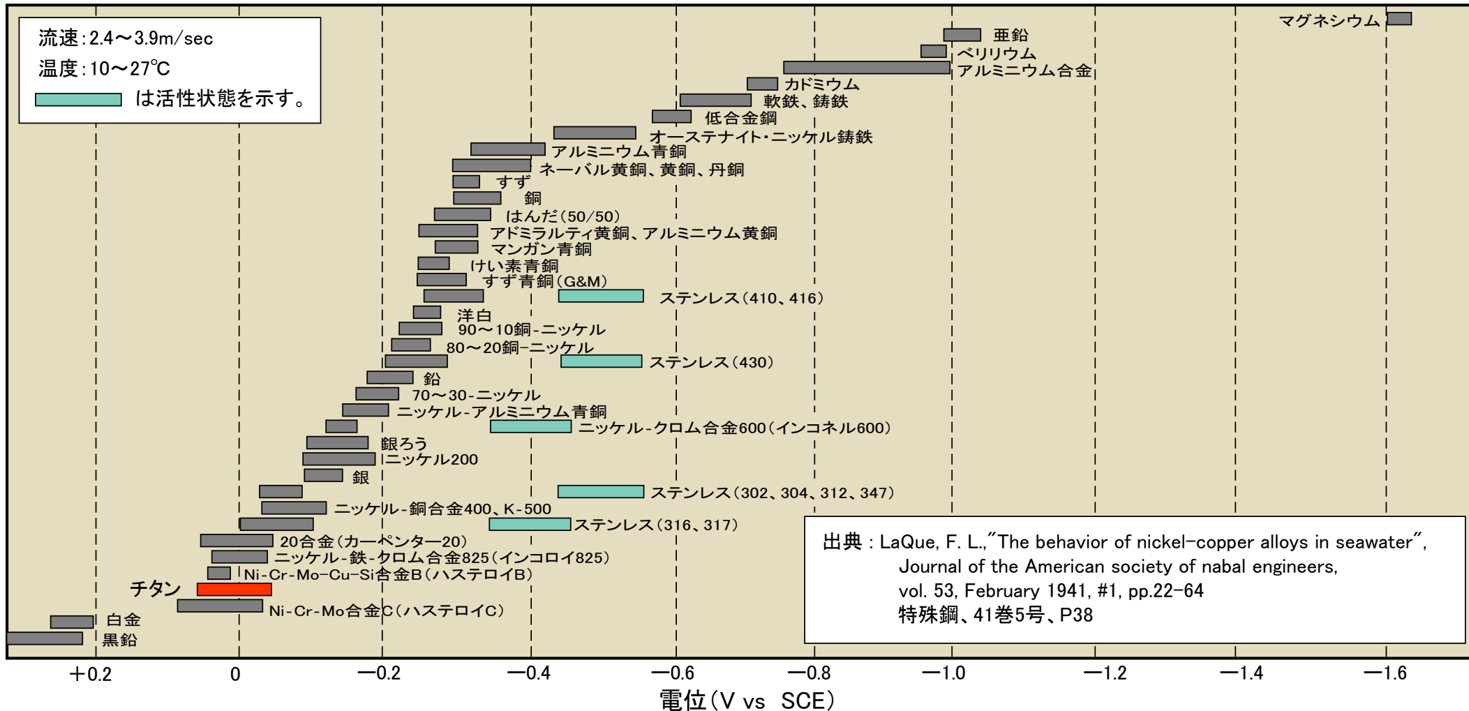
図6.流動海水中における各種金属の自然電位
