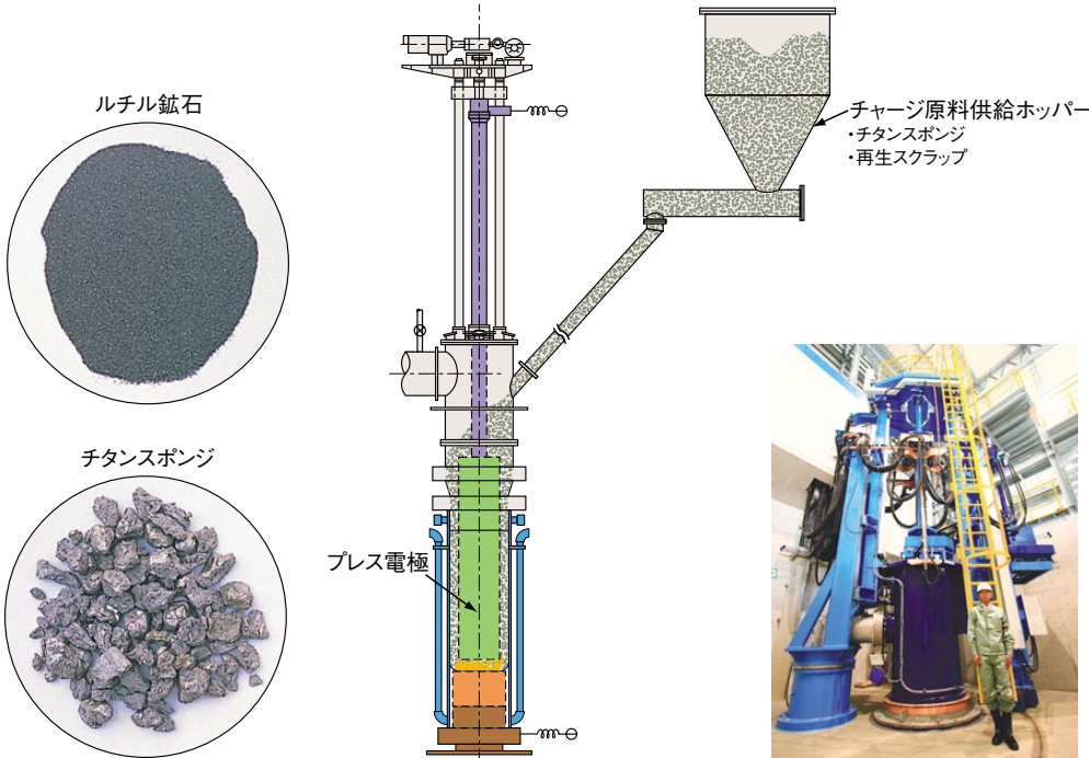
チャージ式溶解炉
