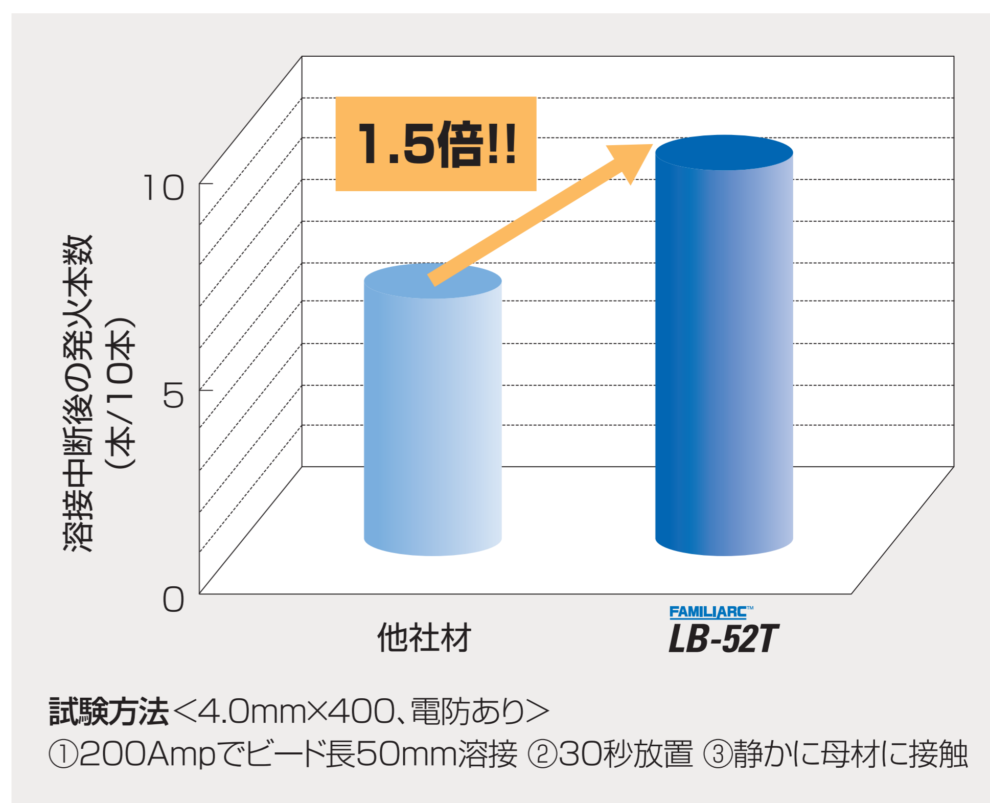
図1 再アーク性の比較
