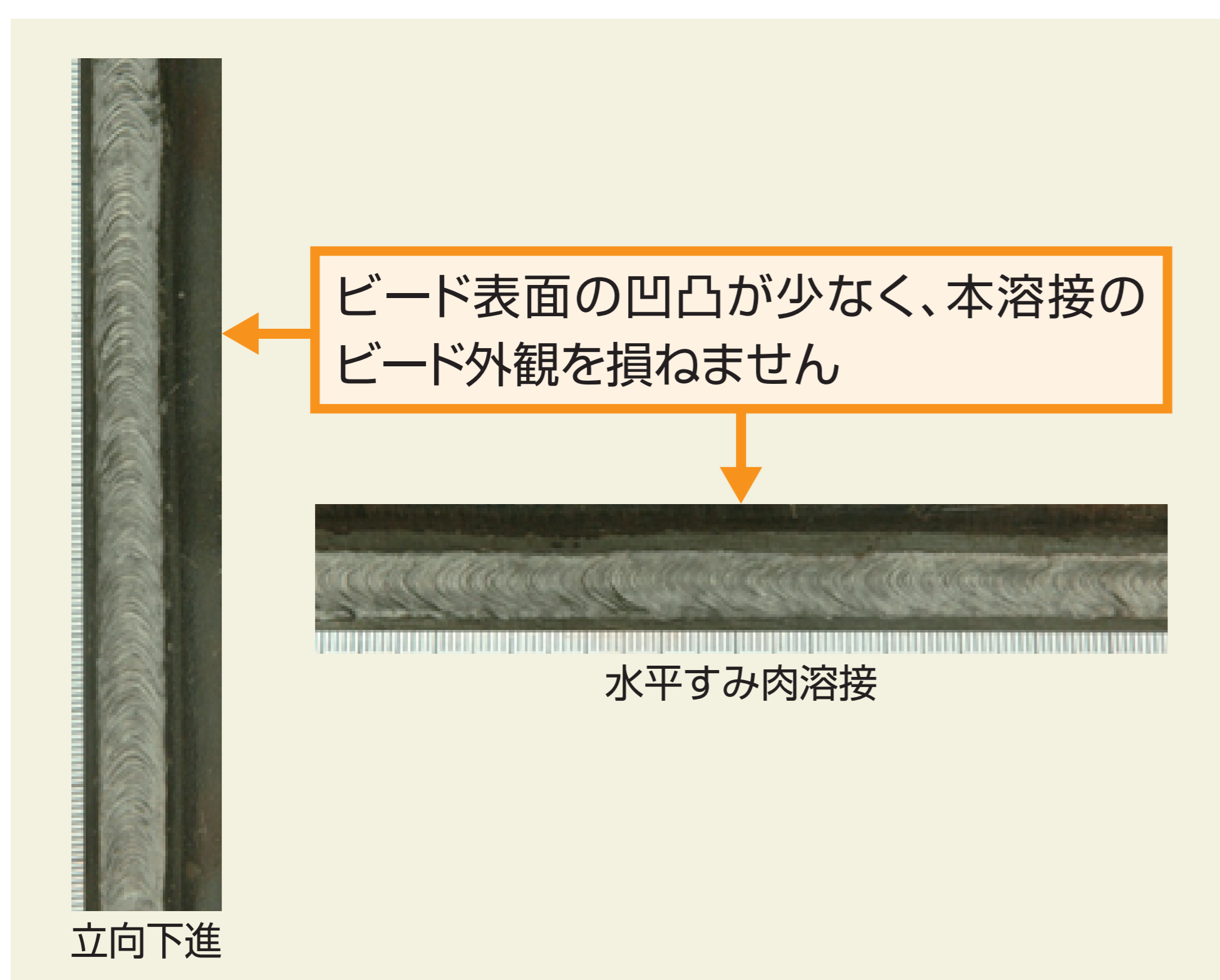
写真1 ビード外観
