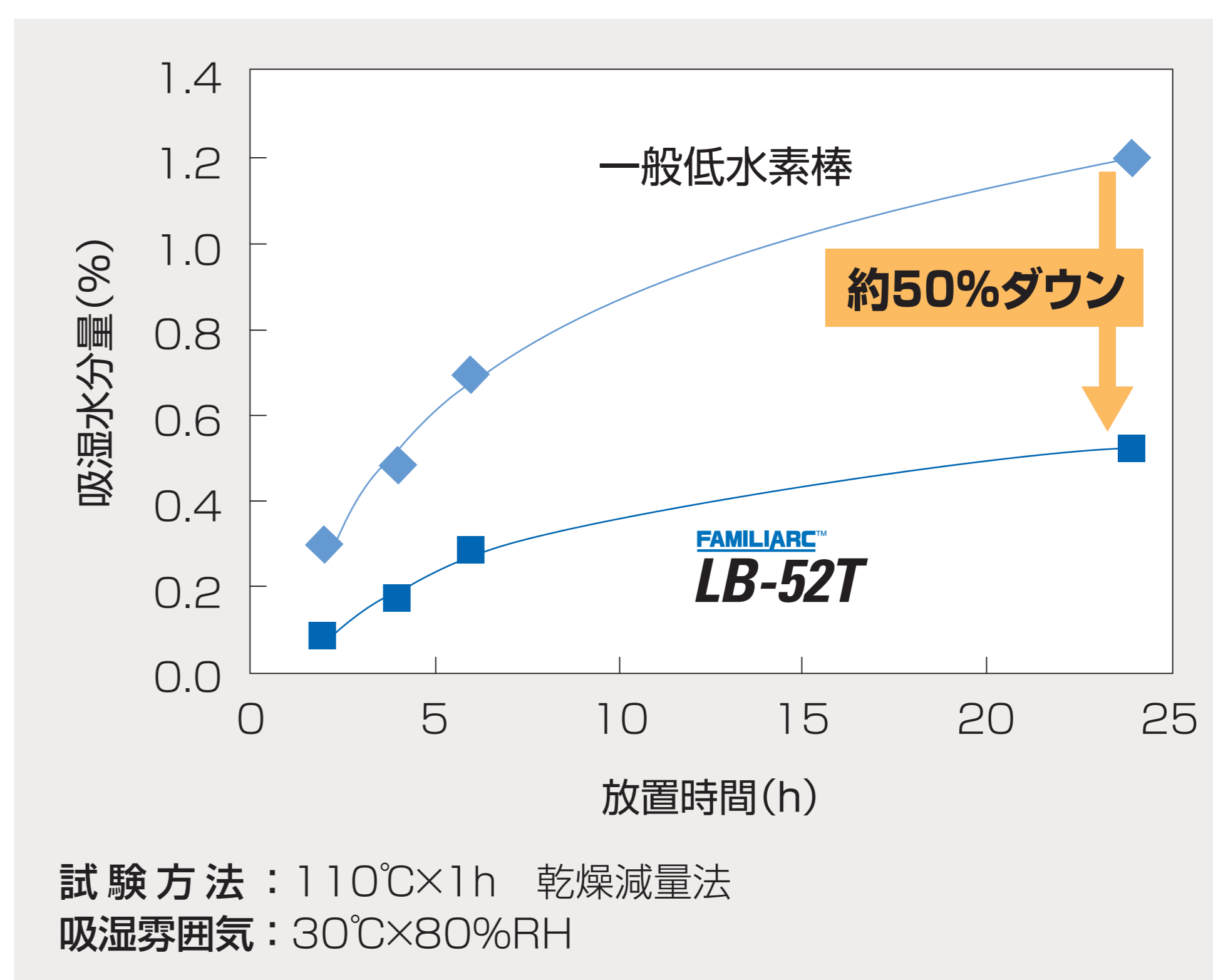
図2 吸湿水分量の比較
