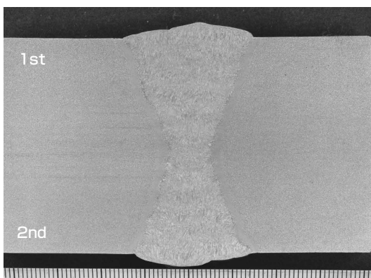
鋼板：K-TEN780 シールドガス：80%Ar-20%CO 2 溶接姿勢：立向上進 溶接条件：200A-24V
