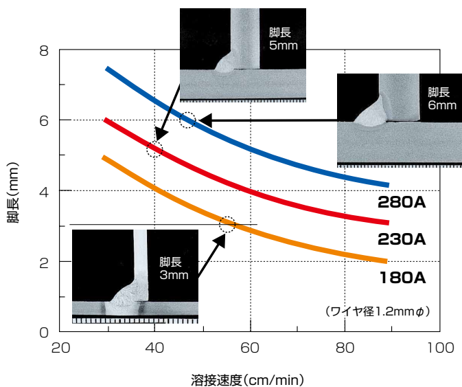
溶接速度と水平すみ肉脚長の関係
