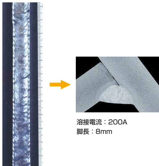
立向上進すみ肉のビード外観と断面マクロの一例
