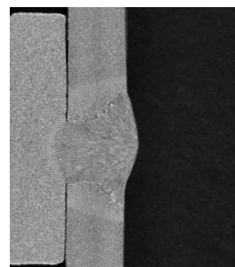
断面マクロ
